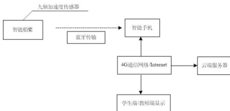
图1 智能龙舟训练系统
